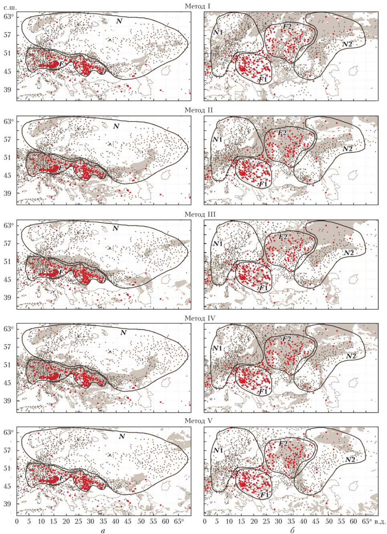
Рис. 1. Карты расчета дальности видимости для прогноза туманов по пяти методам (заштрихованные области) и данные наблюдений за туманами на метеостанциях (красные точки – наличие туманов, черные – их отсутствие): для 06:00 6 февраля 2017 г. (а) и для 06:00 25 октября 2015 г. (б)
