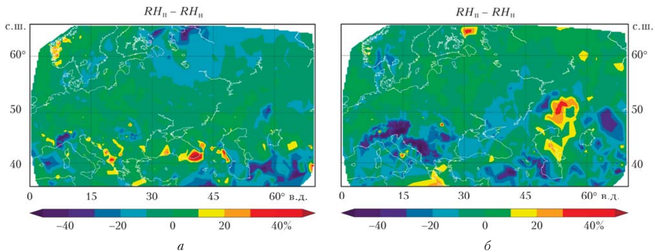
Рис. 2. Карты разности значений относительной влажности на высоте 2 м по данным модели WRF-ARW ( RH_{II} ) и по данным наблюдений на метеостанциях ( RH_{II} ) в 06:00 6 февраля 2017 г. ( a ) и 06:00 25 октября 2015 г. ( б )
