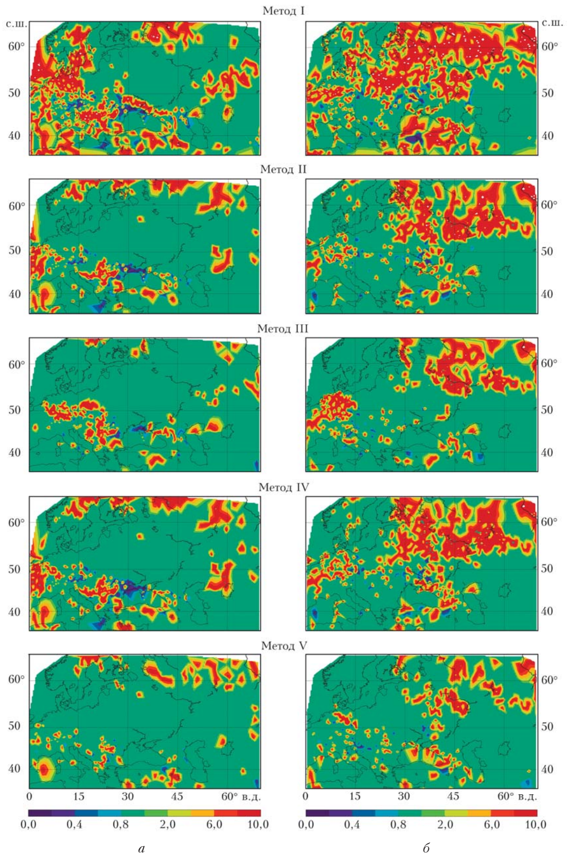
Рис. 3. Карты отношения длительности прогноза тумана по всем пяти методам к длительности тумана по данным наблюдений на синоптических станциях 5–7 февраля 2017 г. ( a ) и 24–26 октября 2015 г. ( б )
