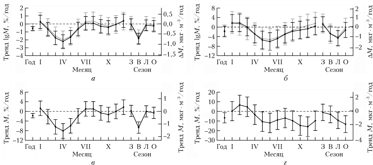
Рис. 5. Годовая (точка слева), месячные (кривые в центральной части) и сезонные (кривые справа) оценки тренда логарифма концентрации аэрозоля (а, б) и концентрации аэрозоля (в, г) и их 95% доверительные интервалы при порядке авторегрессии k = 70 (серый цвет) и k = 400 (черный цвет) в интервалах 1991–2002 (а, в) и 2013–2018 гг. (б, г); объяснение правой вертикальной оси см. в тексте
