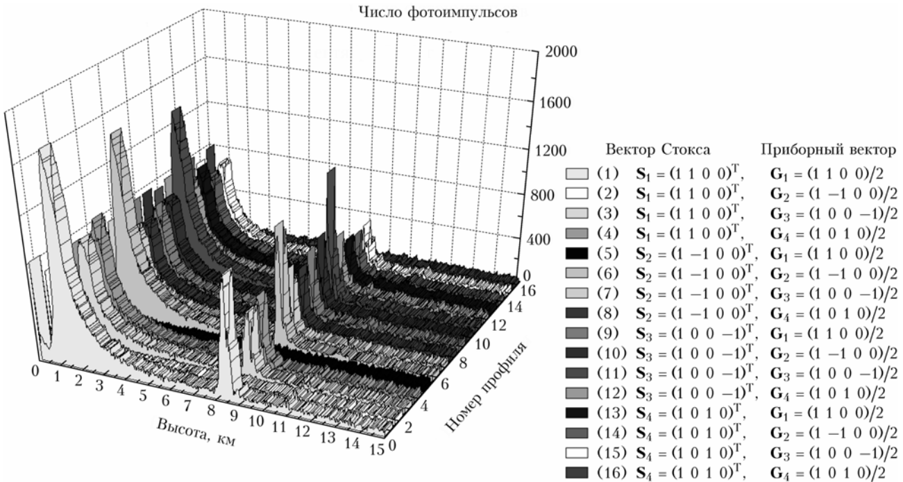
Рис. 4. Вертикальные профили интенсивности обратно рассеянного излучения. 10 сентября 2012 г. Местное время 17:26–17:32
