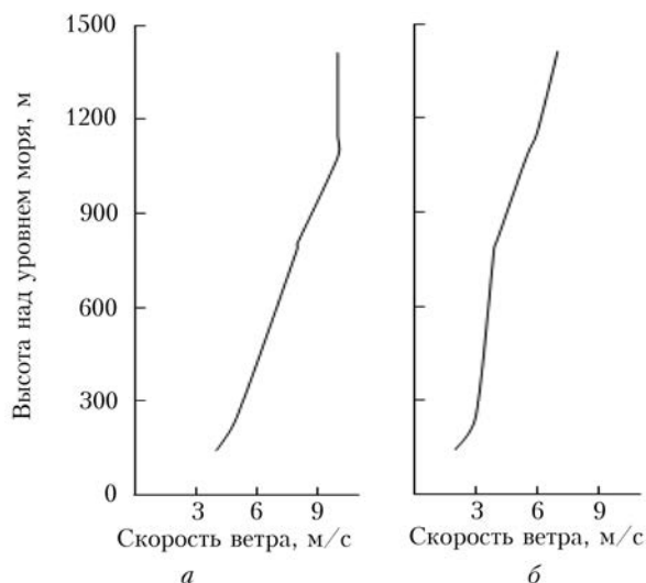
Рис. 3. Распределение скорости ветра с высотой 1 февраля 2019 г. по данным аэрологической станции г. Новосибирска в 00:00 (а) и 12:00 UTC (б)
